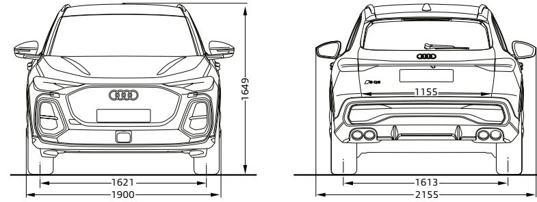
SQ5 SUV
